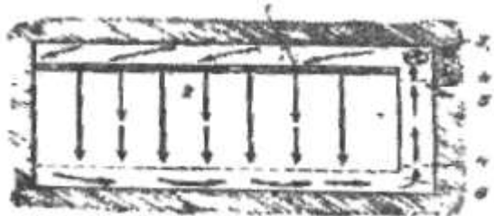
3-rasm. Operatsiya xonasida havoning vertikal oqimi sxemasi. 1-filtr; 2-havo oqimi; 3-ventilyator; 4-filtr oldi qismi; 5-tashqi muhitdan tushuvchi havo; 6-teshik pol
